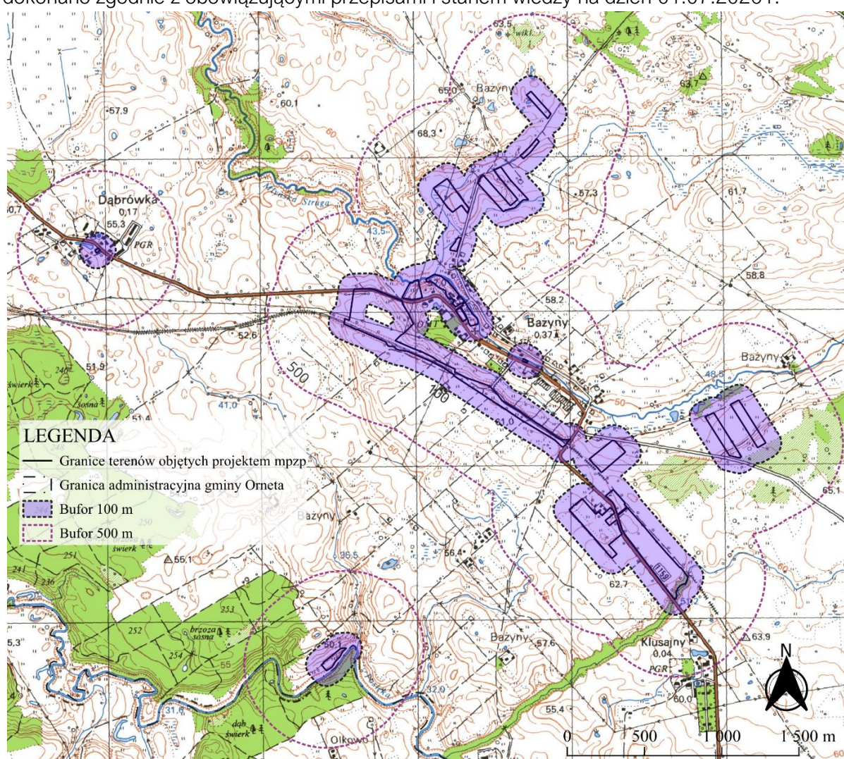
Rysunek 1. Obszar podstawowy objęty analizą porównawczą Źródło: Qgis, opracowanie własne na mapie topograficznej
