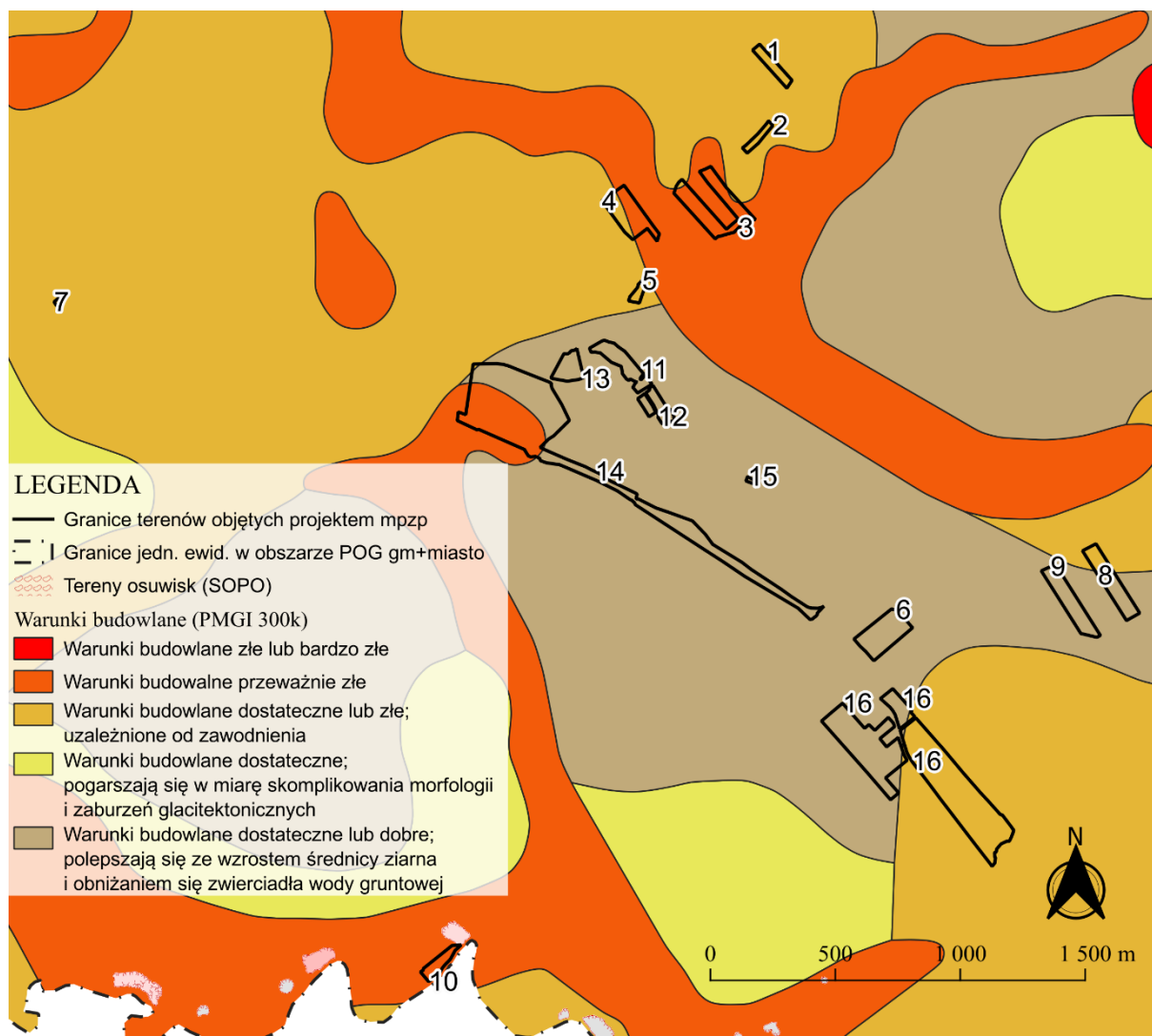
Rysunek 13. Obszar planu na tle warunków budowlanych wg Państwowej Mapy Geologiczno-Inżynierskiej
