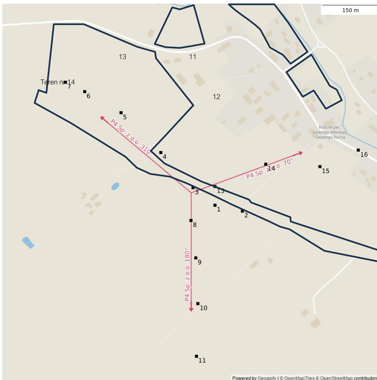
Rysunek 16. Lokalizacja pionów pomiarowych w miejscowości Bążyny na tle fragmentu planu
